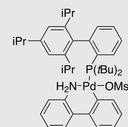
t-BuXPhos Pd G3
