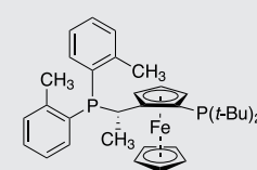
Josiphos
