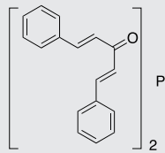
Pd(dba) 2
