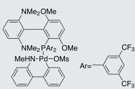
SPhos Pd G4
