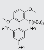
t-butylBrettPhos SC-5017 1160861-53-9
