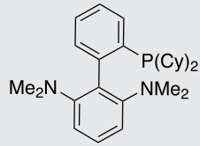
Cphos SC-5021 1160556-64-8
