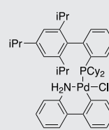
XPhos Pd G2
