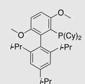
BrettPhos SC-5018 1070663-78-3
