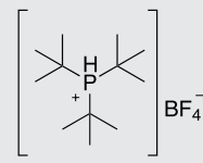
(t-Bu) 3 PHBF 4
