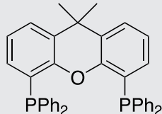
XantPhos
