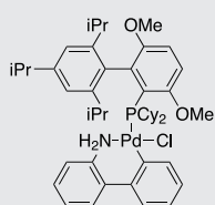
BrettPhos Pd G2
