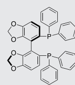
(R)-(+)-SEGPPOS
