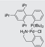
t-BuXPhos Pd G1 SC-5034 1142811-12-8
