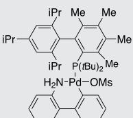
Me4 t-ButylXPhos Pd G3
