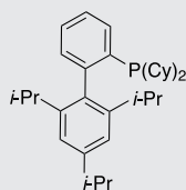
XPhos SC-5002 564483-18-7
