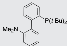
tBuDavePhos SC-5005 224311-49-3
