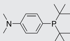
A-taPhos
