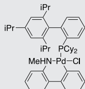
XPhos Pd G4
