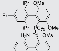
BrettPhos Pd G3
