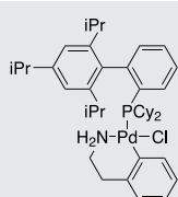
XPhos Pd G1 SC-5033 1028206-56-5
