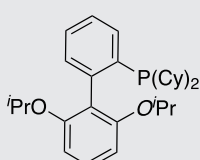
RuPhos SC-5011 787618-22-8
