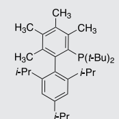
Me 4 t-butylXPhos SC-5013 857356-94-6
