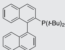
TrixiePhos SC-5010 255836-67-0
