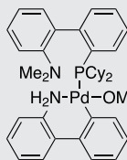
DavePhos Pd G3
