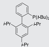
tBuXPhos SC-5003 564483-19-8
