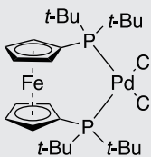
Pd(DtBPF)Cl 2
