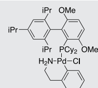
BrettPhos Pd G1 SC-5035 1148148-01-9
