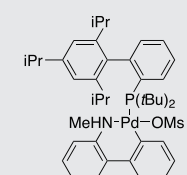
t-BuXphos Pd G4
