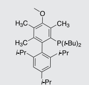
Me 3 (OMe)tBuXPhos SC-5019 1359986-21-2
