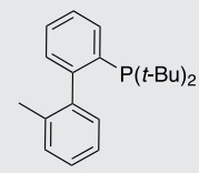
tBuMePhos SC-5009 255837-19-5
