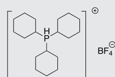
PCy 3 HBF 4
