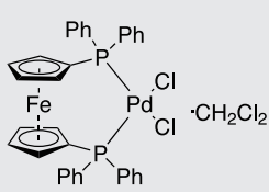
Pd(DPPF)Cl 2 · CH 2 Cl 2
