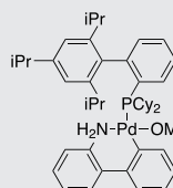
XPhos Pd G3
