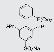
XPhos-SO 3 Na SC-5014 870245-84-4
