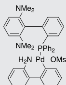
PhCphos Pd G3
