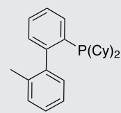
MePhos SC-5008 251320-86-2
