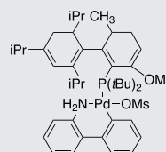
RockPhos Pd G3
