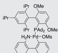
AdBrettPhos Pd G3
