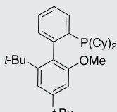
VPhos SC-5027 1848244-75-6
