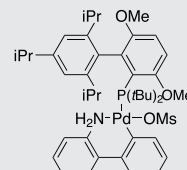
t-butylBrettPhos Pd G3
