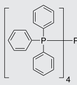
Pd(PPh 3 ) 4
