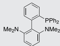
PhCPhos SC-5029 1447963-71-4
