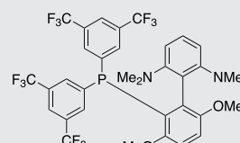
t-BuXPhos Pd G1 SC-5026 1810068-30-4
