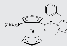
Josiphos
