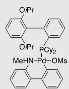
RuPhos Pd G4
